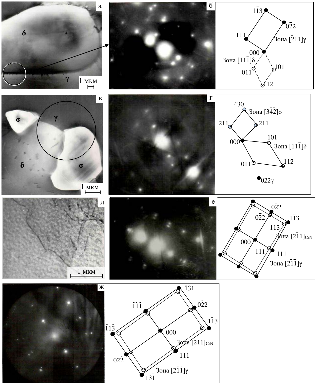
Рис. 37 – Сталь 05X22AГ15Н8М2ФЛ после отжига 1100 °С, 1 ч: а– типичный участок структуры с \delta -ферритом, б – микродифракции с участка на рис. «а» и схемы её расшифровки; в– частицы \sigma -фазы на границе \gamma/\delta , г – микродифракции от участков структуры на рис. «в» и схема её расшифровки д – субструктура аустенита, е – микродифракция с участка на рис. «д» и схема её расшифровки [2\bar{1}\bar{1}]\gamma // [2\bar{1}\bar{1}]_{\text{CrN}} ; ж – электроннограмма в режиме электронографа [2\bar{1}\bar{1}]\gamma // [2\bar{1}\bar{1}]_{\text{CrN}} ;
