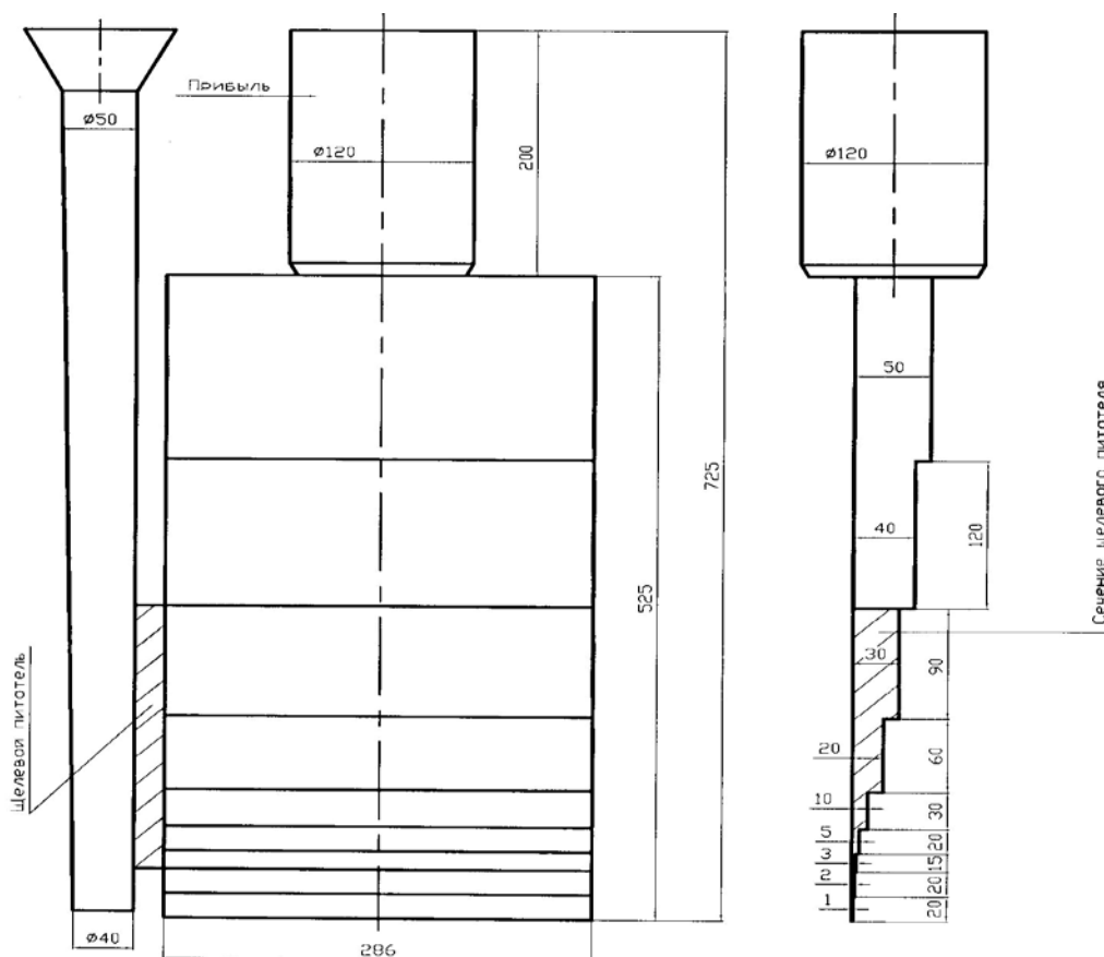
Рис. 12 – Эскиз модельной отливки из стали 05X22AG15H8M2ФЛ.
