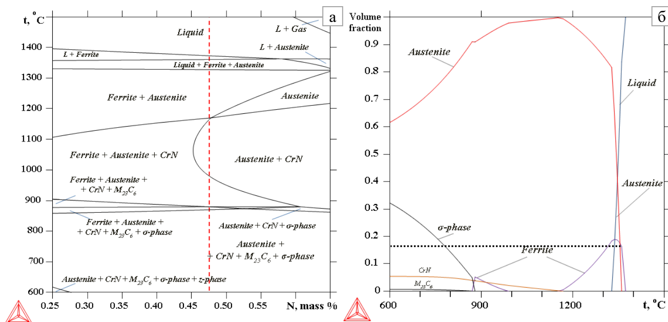
Рис. 16 – Расчёты термодинамически равновесного фазового состава для исследованной стали: а - фазовая диаграмма для изученной стали при содержании азота от 0,25 до 0,65 масс.%; - - - - - содержание азота в исследованной стали; б - объемная доля фаз в стали в интервале температур 600 – 1500°C; ..... – количество \delta -феррита, образовавшегося в жидкой фазе до начала образования кристаллов аустенита
